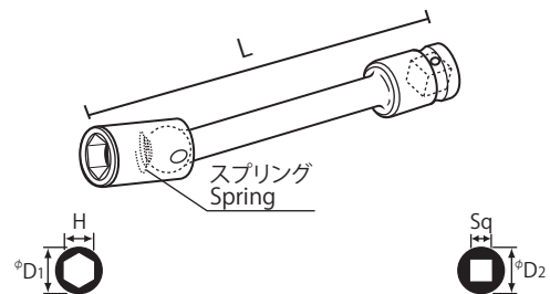
12.7Sq. ユニバーサルソケット (エクステンションタイプ) Universal Extension Sockets (Single Hex)
